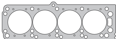
25090AM1 / MLS NO SE INCLUYE EN JUEGO DE JUNTAS
